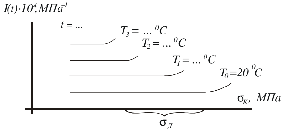
Рис. 2.1.3. Визначення областей лінійності в'язко-пружних властивостей матеріалів за залежностями I - \sigma_K при фіксованому часі спостережень t та різних температурах T .
