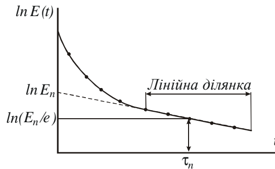
Рис 2.5.1. Схема визначення E_n та \tau_n
