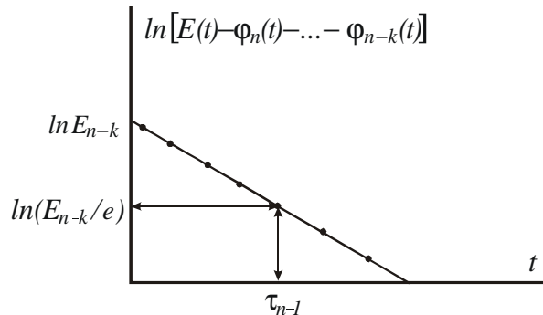
Рис. 2.5.3. Схема визначення E_{n-k} та \tau_{n-k} (останній крок)
