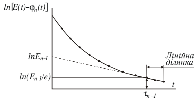
Рис 2.5.2. Схема визначення E_{n-1} та \tau_{n-1}
