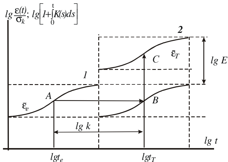
Рис 2.4.1 Схема визначення параметрів ядра рівняння повзучості.
