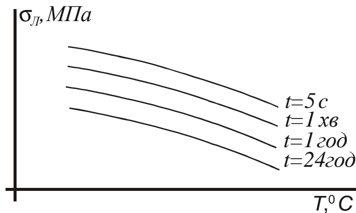
Рис. 2.1.4. Залежності межі лінійні в'язкопружності \sigma_L від температури випробувань T .
