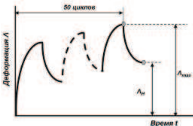
Рис. 5. Обработка кривых циклического деформирования (измерение максимальных \Delta_{max} и необратимых \Delta_n деформаций)
